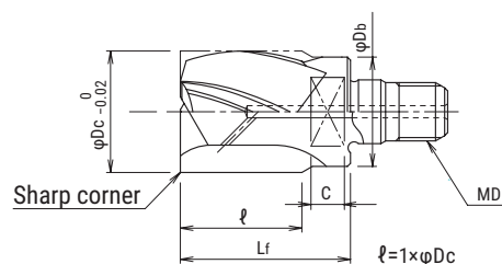
Helix angle 45°
