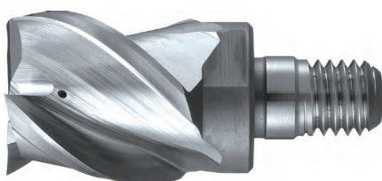
Helix angle 45°
