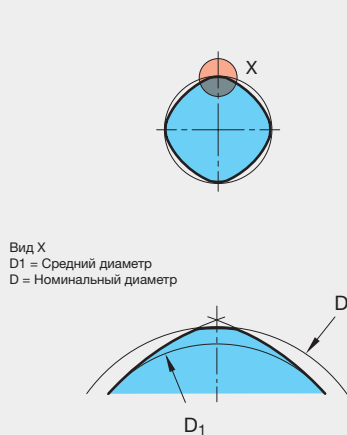
Радиальное сечение бесстружечного метчика
