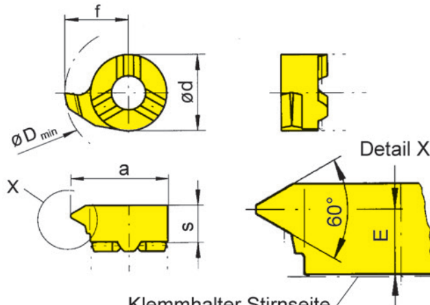
Klemmhalter Stirnseite Toolholder face
