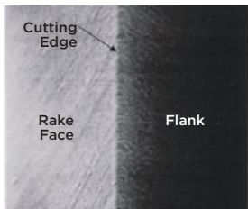
UPC cutting edge
