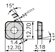
Fig 1 (材質ACP/ACKシリーズの場合) Fig 2
