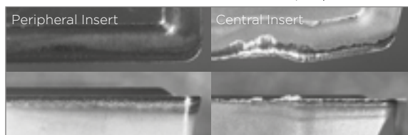
Rake face wear/fracture
