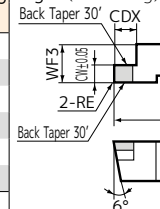
Fig 1 (Grooving)
