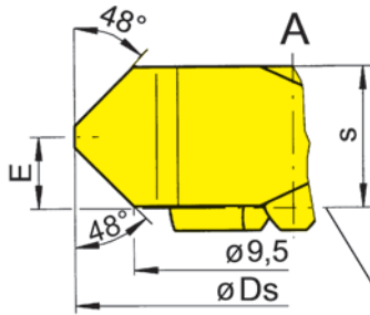
Fräaserschaft Milling shank
