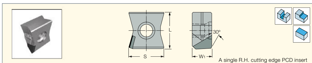
A single R.H. cutting edge PCD insert
