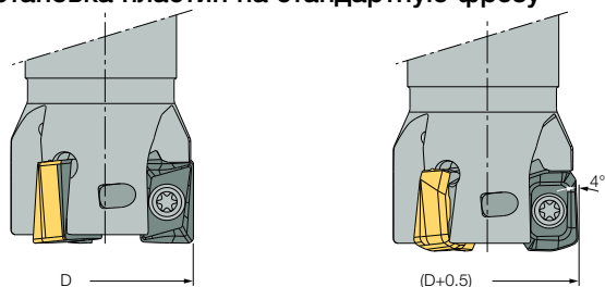
Фреза с обычными пластинами
