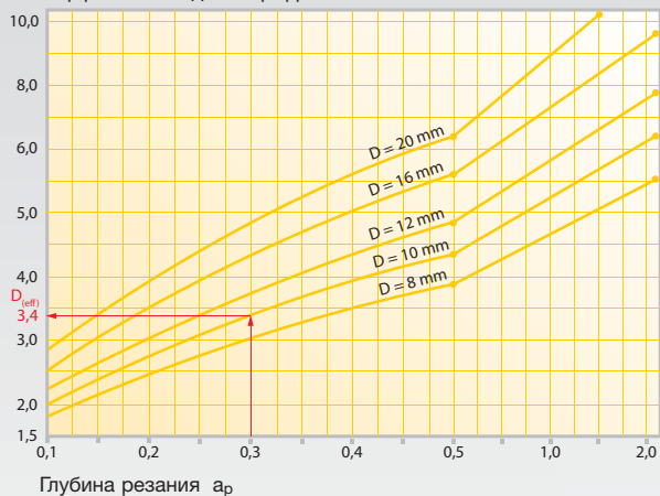
Эффективный диаметр фрезы
