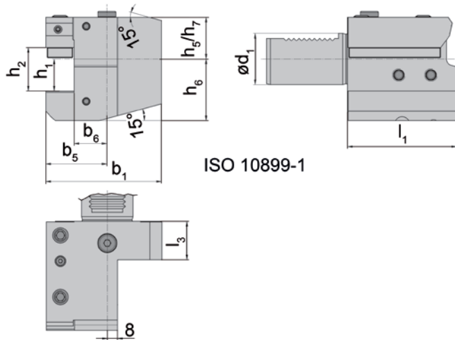
Abbildung = VDI-Halter Typ C2
